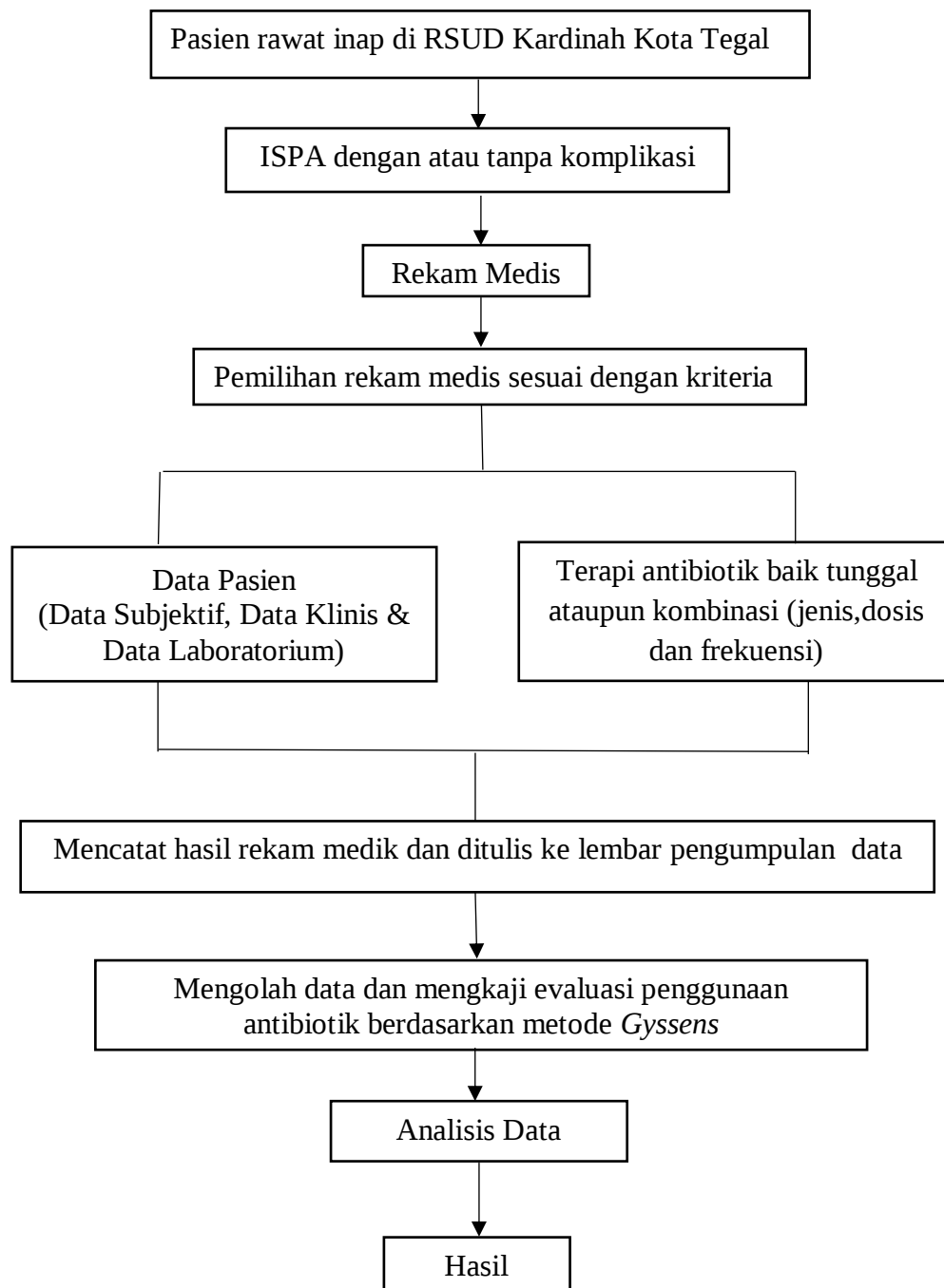
Gambar 3.1 Rancangan Penelitian
